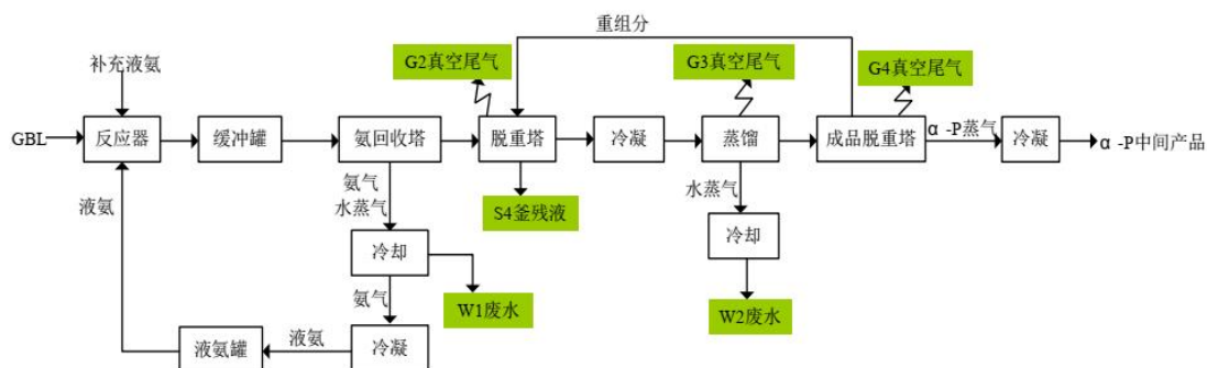
图 4-8 α-p 生产工艺流程及产污环节图
