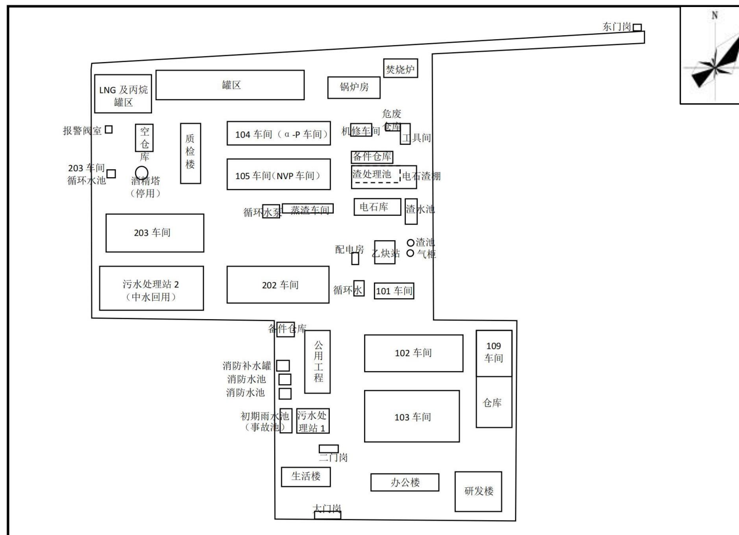
图 4-17 厂区平面布置图
